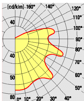
Sijalka – mešana svetloba
