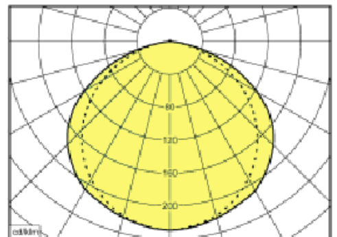
Diagram svetilnosti -2 sijalke Izkoristek: 72 %
